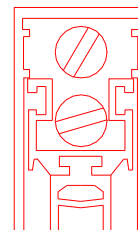
Figura 6 Guarnizione a ghigliottina inferiore
